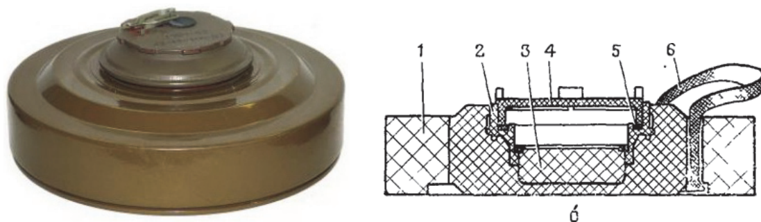
Рис. 7.2. Противотанковая мина ТМ-62М с взрывателем МВЧ-62: а – общий вид мины со взрывателем; б – разрез мины; 1 – заряд; 2 – стакан; 3 – дополнительный детонатор; 4 – пробка; 5 – прокладка; 6 – ручка
