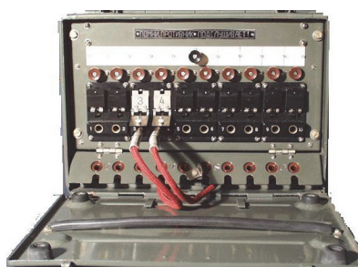
Рис. 6.8. Полевой телефонный коммутатор П-193
