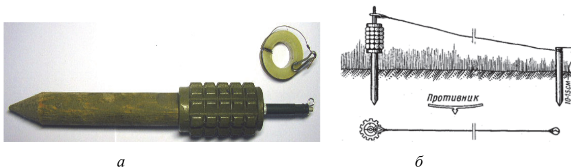
Рис. 7.6. Противопехотная осколочная мина ПОМЗ-2М: а – общий вид мины; б – схема установки мины
