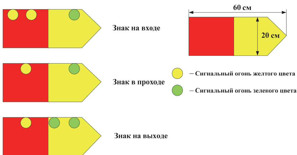
Рис. 7.9. Стандартные указатели для обозначения прохода
