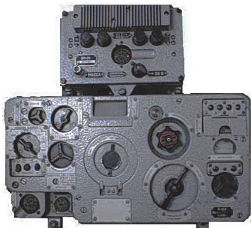
Рис. 6.3. Радиостанция Р-123М
